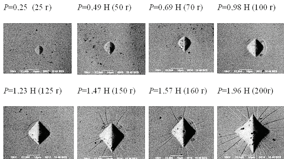
Рис. 3. РЕМ-картини деформацій поверхні аморфного сплаву \text{Fe}_{73,6}\text{Si}_{15,8}\text{B}_{7,2}\text{Cu}_{1,0}\text{Nb}_{2,4} , які виникають навколо відбитків алмазного індентора Віккерса за різних навантажень.
